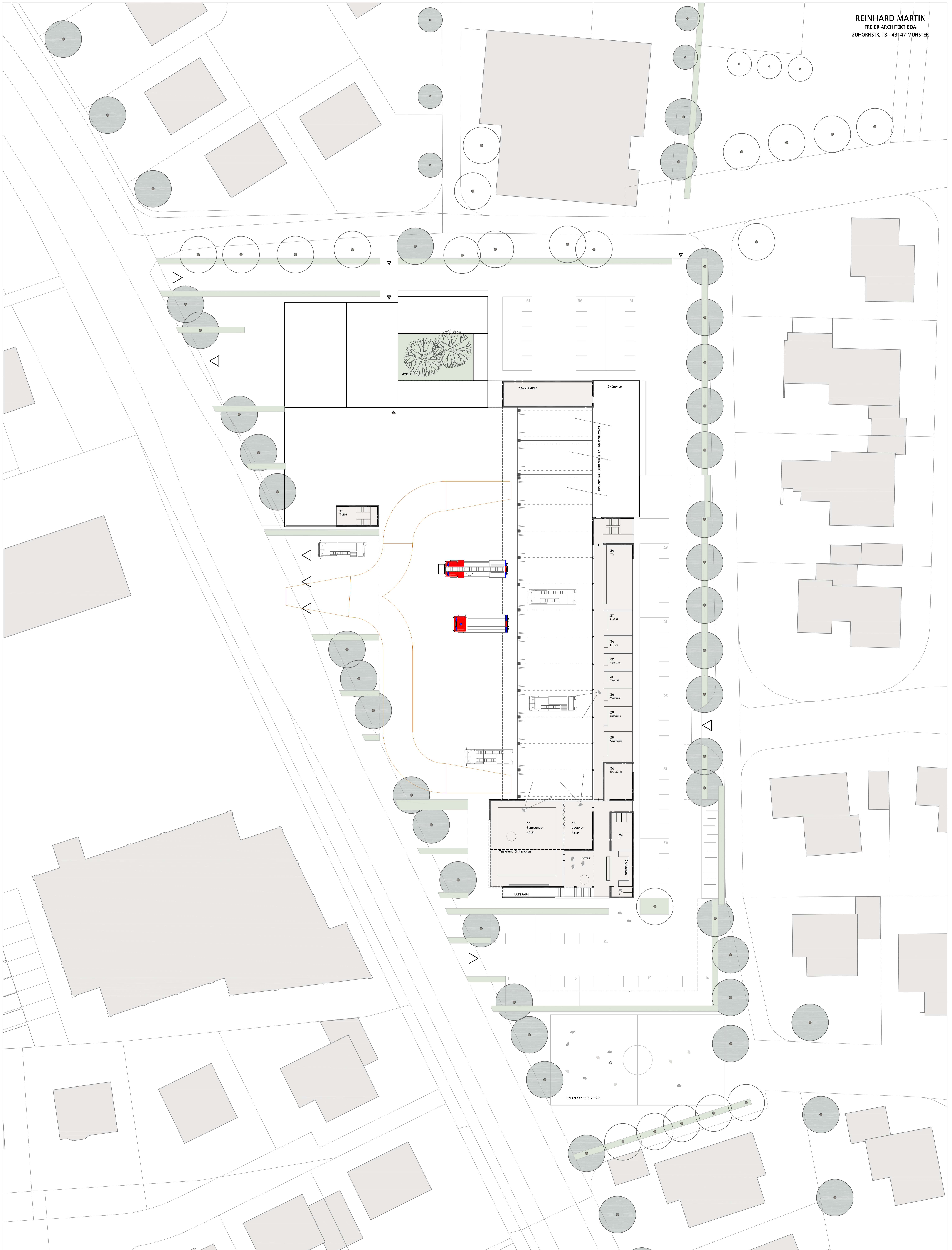
2. PHASE FEUERWEHRGERÄTEHAUS UND RETTUNGSWACHE TELGTE - OG 1:200
